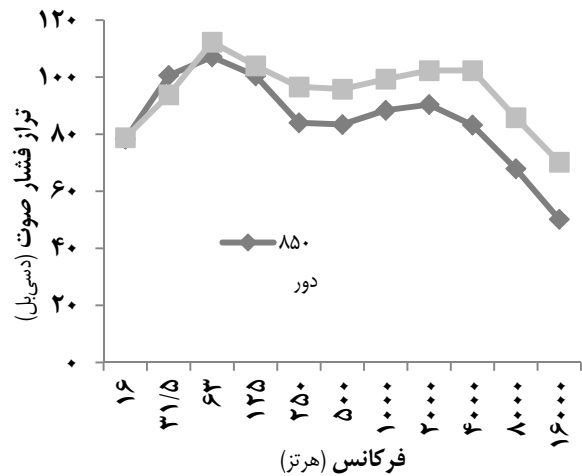
نمودار ۱) نتایج آنالیز فرکانس در موقعیت خروجی اگزوز تراکتور رومانی (م-۶۵۰) در حالت ثابت در دور موتورهای انتخابی
